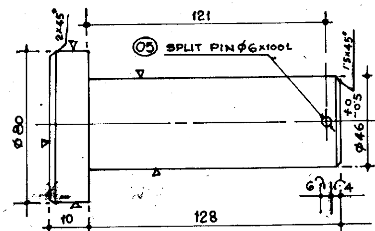
PIN ITEM. 03
