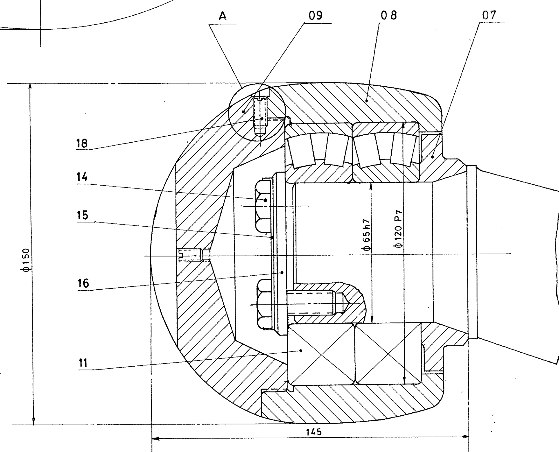
SECTION A-A SCALE: 1:1
